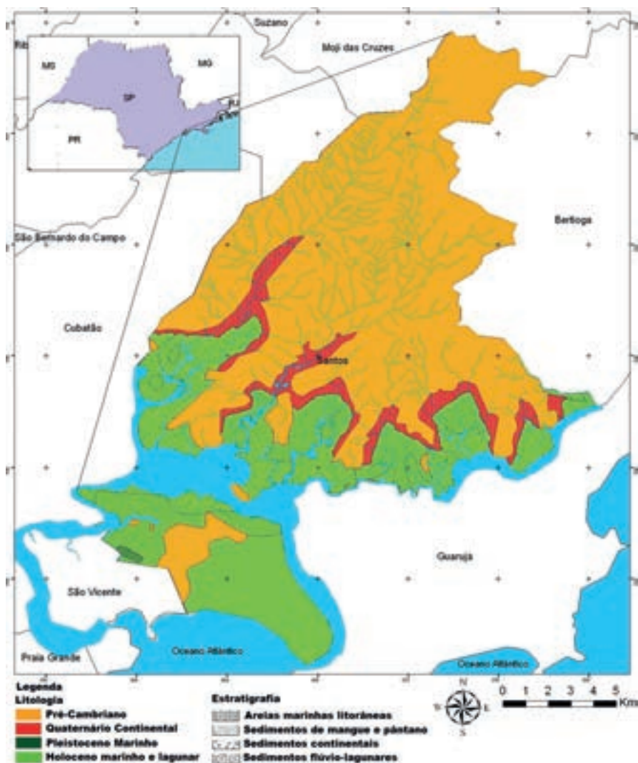
Figura 4.7. Carta Geológica
